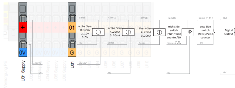
Wire U1/U2
